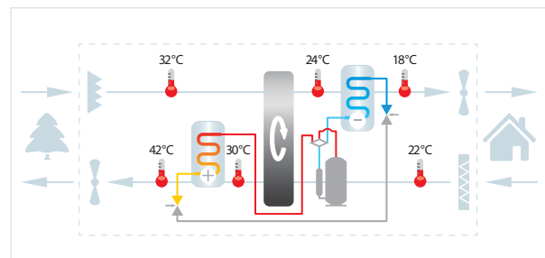
Lüftung mit Wärmerückgewinnung und Luftkühlung
