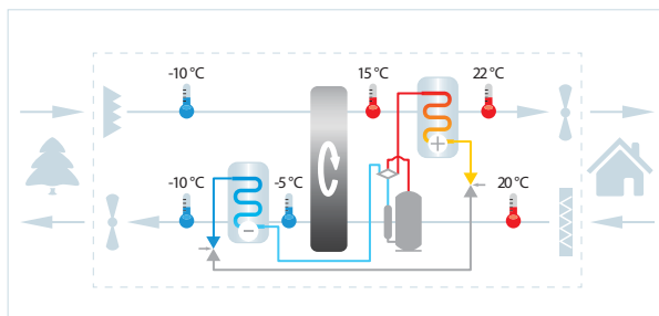
Lüftung mit Wärmerückgewinnung und Luftvorheizung
