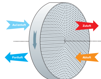
Wirkungsweise des Rotationswärmetauschers
