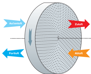
Wirkungsweise des Rotationswärmetauschers
